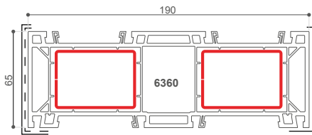
Telaio
