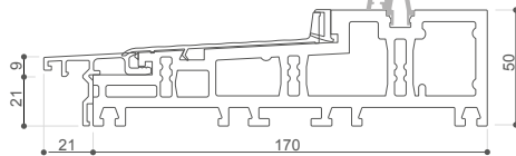
Soglia T.T.
