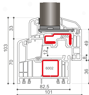
Telaio - Anta
