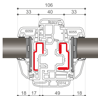
Nodo Centrale 2 ante
