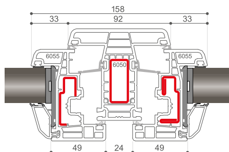
Nodo Anta - Traverso - Anta
