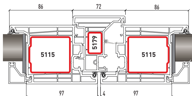
SEZIONE B
