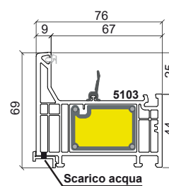
Particolare Telaio con Bancalino
