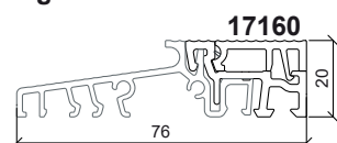
Soglia ribassata DEK-TT
