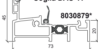
Soglia DAU-TT*
