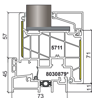
Sezione C Soglia - Anta semimaggiolata
