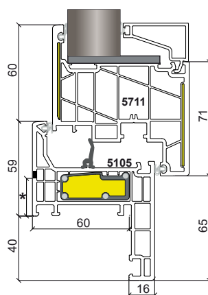
Sezione A - C Telaio - Anta semimaggiorata
