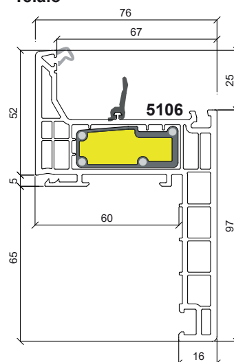
Telaio
