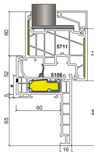
Particolare Telaio con Bancalino
