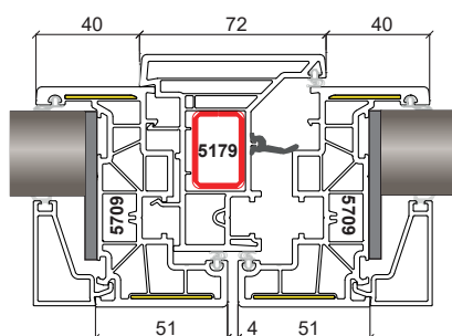
Sezione B Nodo Centrale 2 ante
