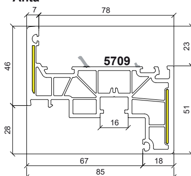
Anta
