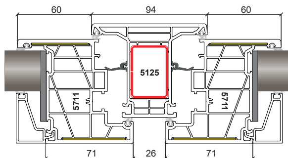
Sezione D Nodo Anta - Trasverso - Anta
