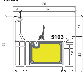
Telaio
