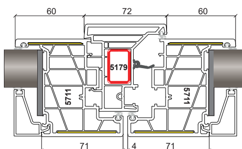
Sezione B Nodo Centrale 2 ante
