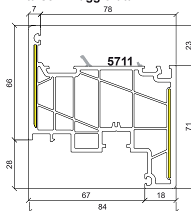
Anta semimaggiorata
