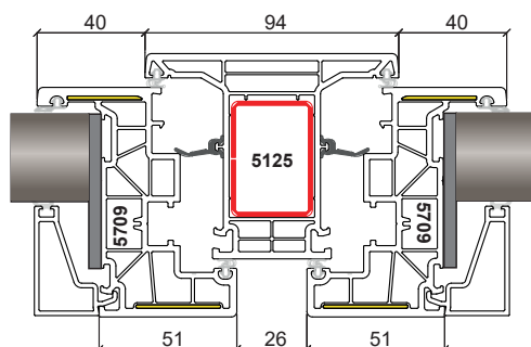
Sezione C Soglia - Anta
