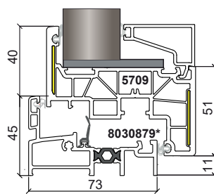
Sezione C Soglia - Anta semimaggiolata
