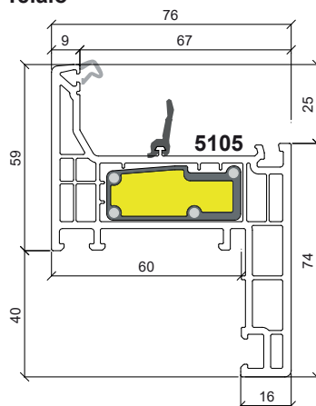
Telaio
