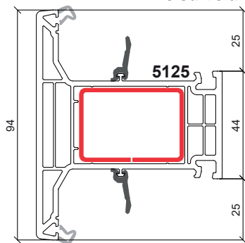
Traverso/Montante su Telaio
