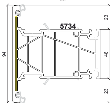
Traverso su Anta
