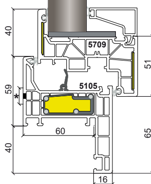
Sezione A - C Telaio - Anta semimaggiorata
