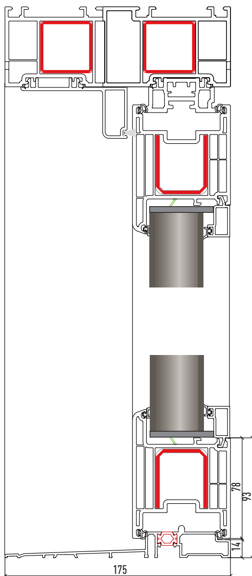
Sezione B-B'
