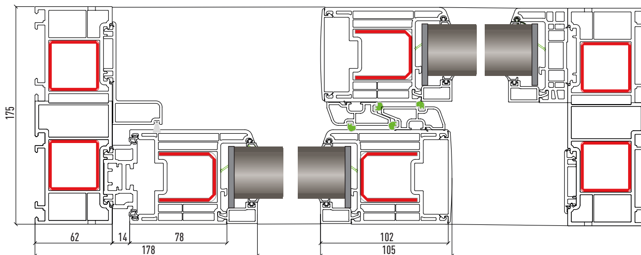
Sezione A-A'
