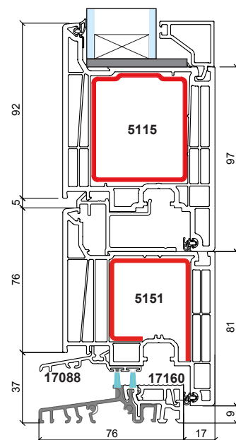
SECTION A-C
